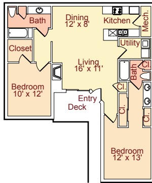
Plan C • 1098 sq.ft.*
