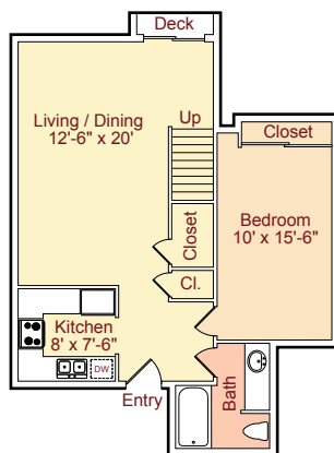
Plan E • 1471 sq.ft.*
